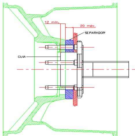
FIG. 6. (medidas en mm)
